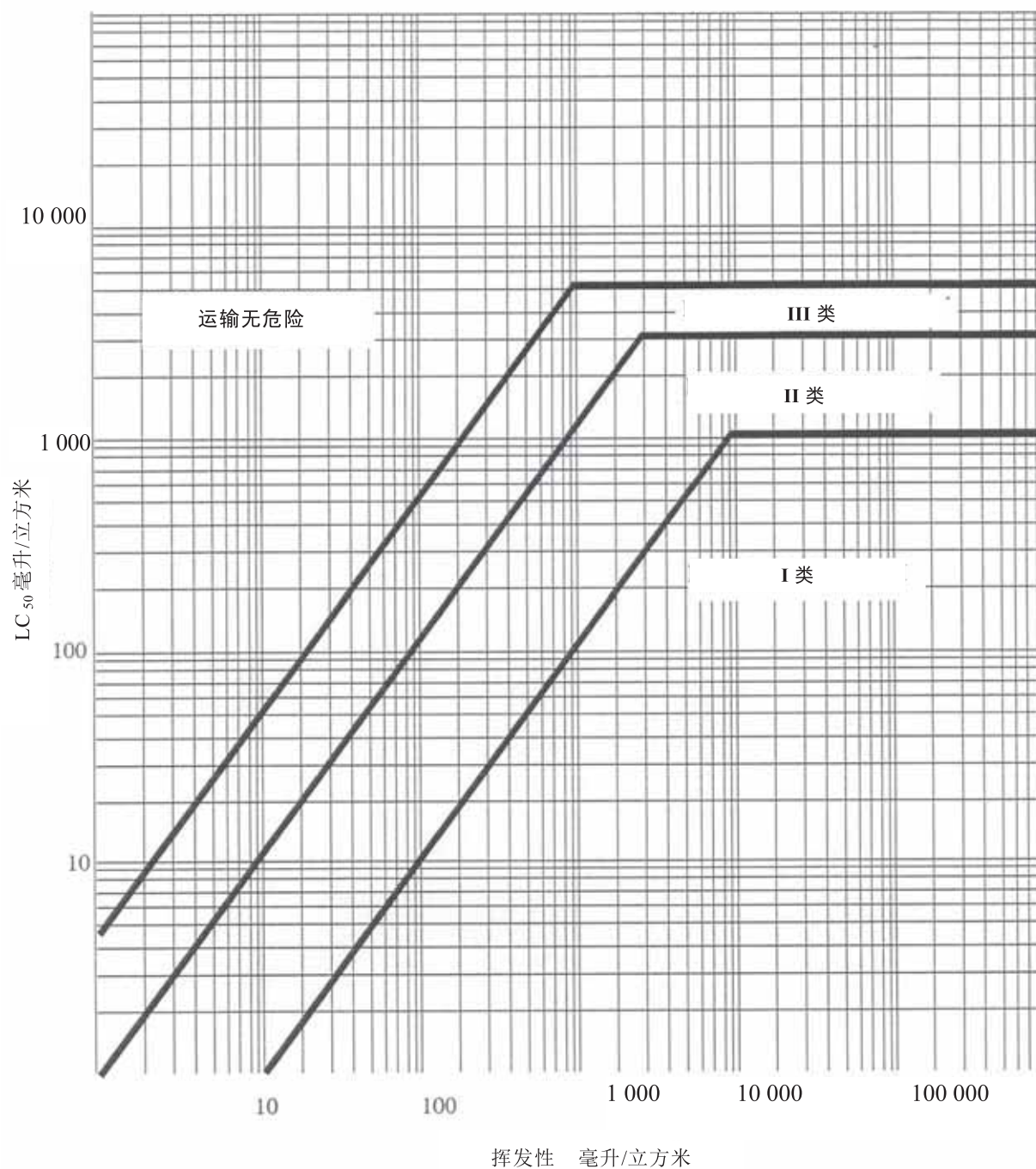
图 2.6.1：吸入毒性：包装类别界线
