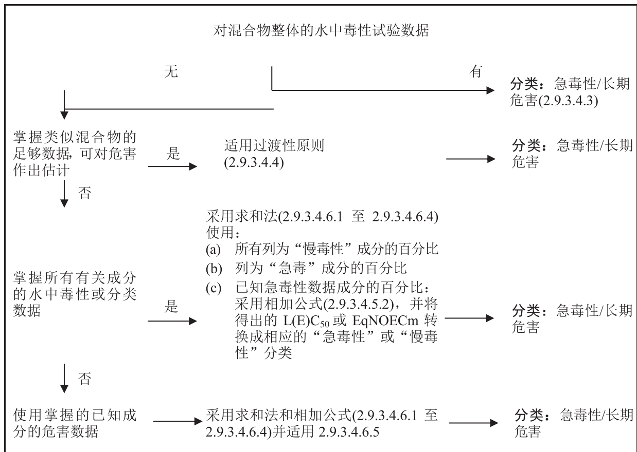
图 2.9.2：采用分层办法对造成急性和长期水生环境危害的混合物进行分类
