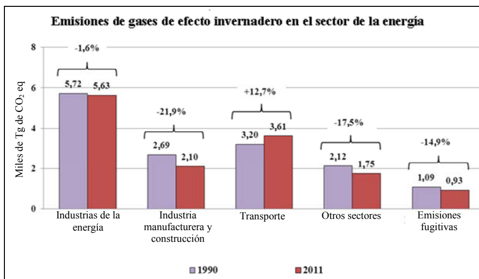
Gráfico 6 Emisiones de gases de efecto invernadero de las Partes del anexo I en el sector de la energía, 1990 y 2011
