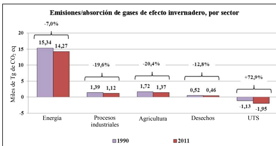
Gráfico 5 Emisiones y absorción de gases de efecto invernadero de las Partes del anexo I por sector, 1990 y 2011 a
