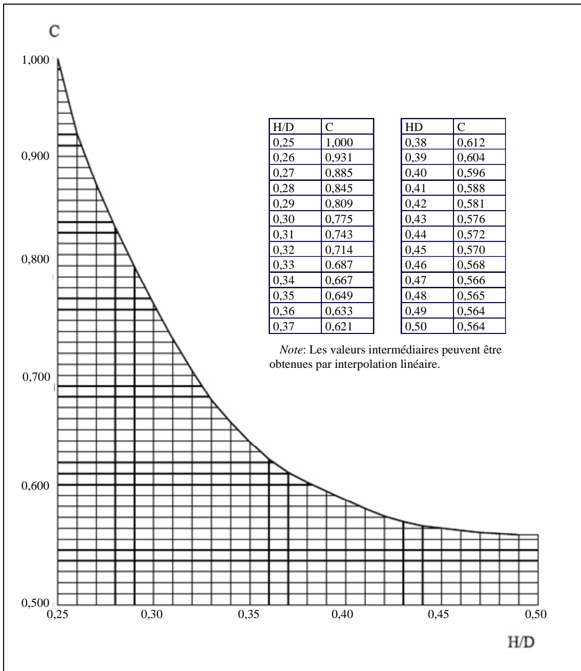
Valeur du coefficient C pour les rapports H/D, de 0,25 à 0,50.
