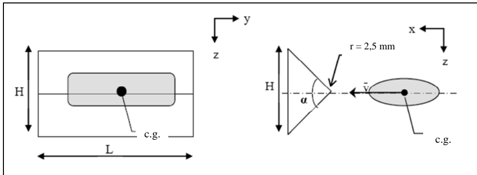
Figure 1 Agencement d'essai
