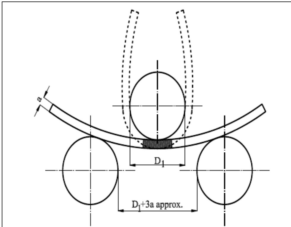
Figure 1 Exemple d'essai de pliage
