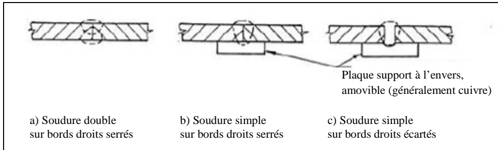
Figure 1 Principaux types de soudures longitudinales bout à bout
