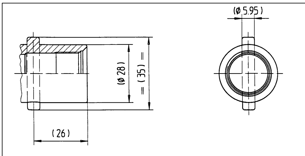
Connecteur de l'embout de remplissage à baïonnette
