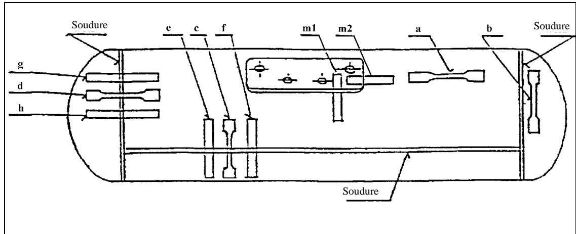
Figure 1 Réservoirs à soudures longitudinales et circulaires, emplacement des éprouvettes
