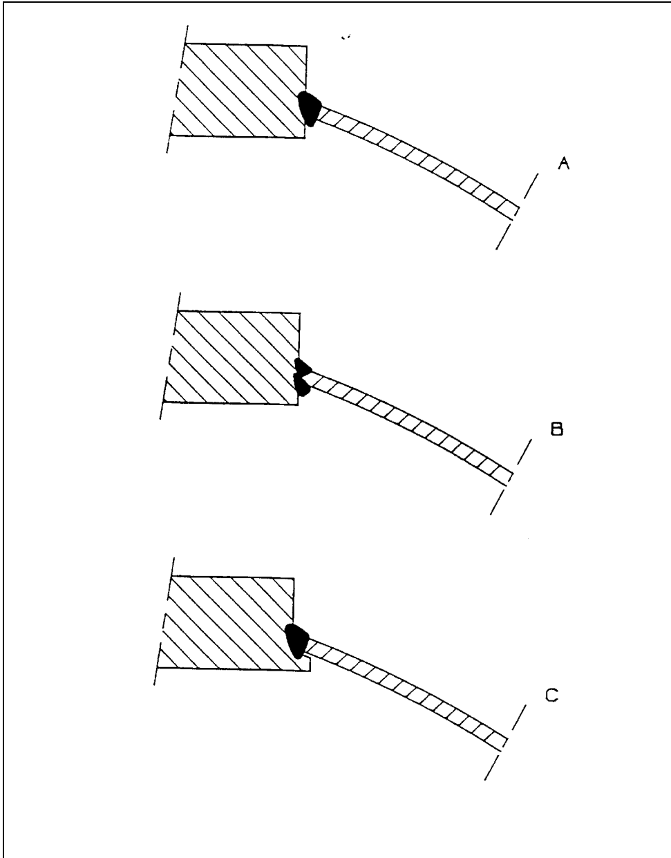
Figure 3 Exemples d'embases à goujons soudées
