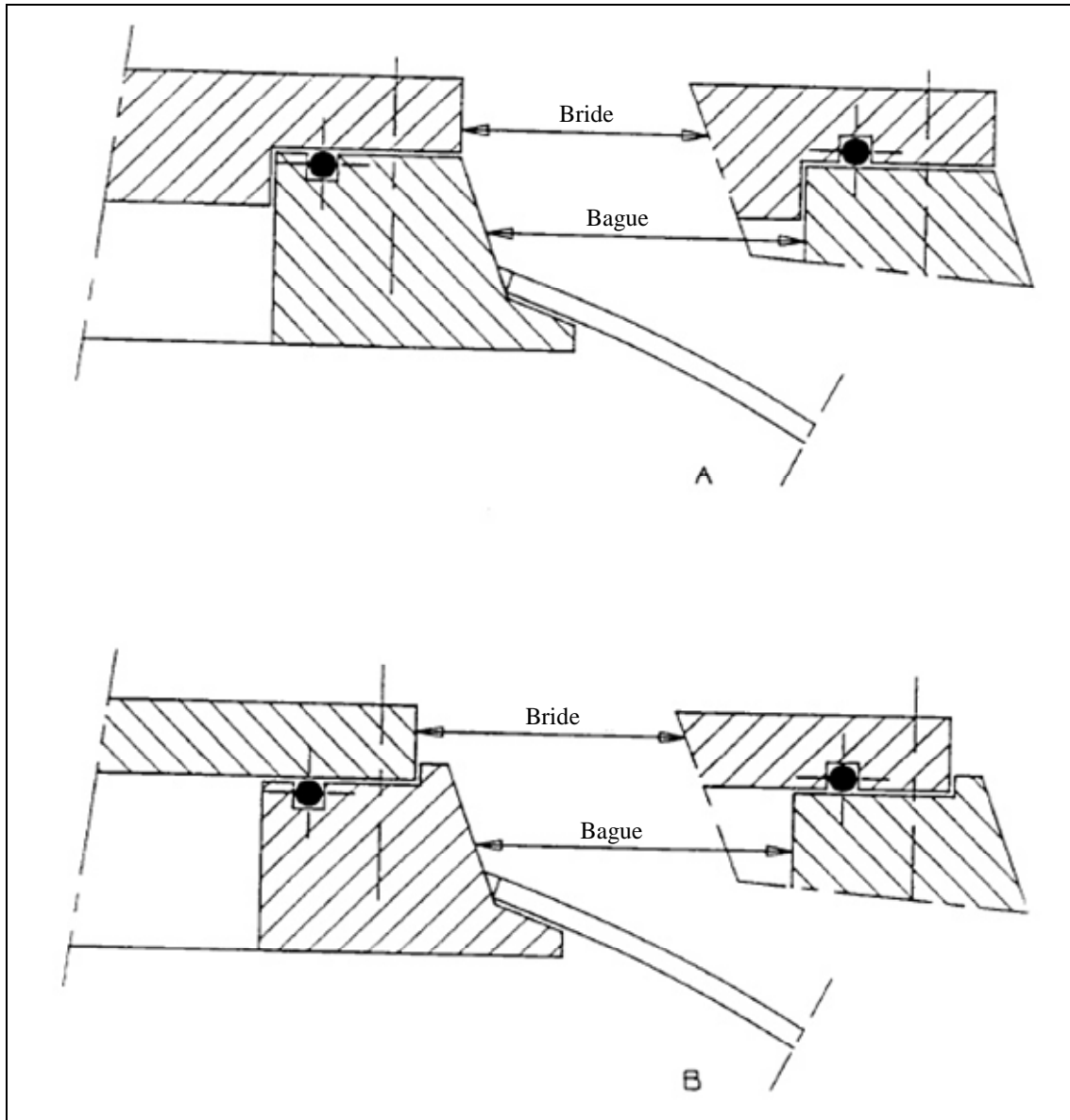
Figure 4 Exemples de bagues soudées avec bride
