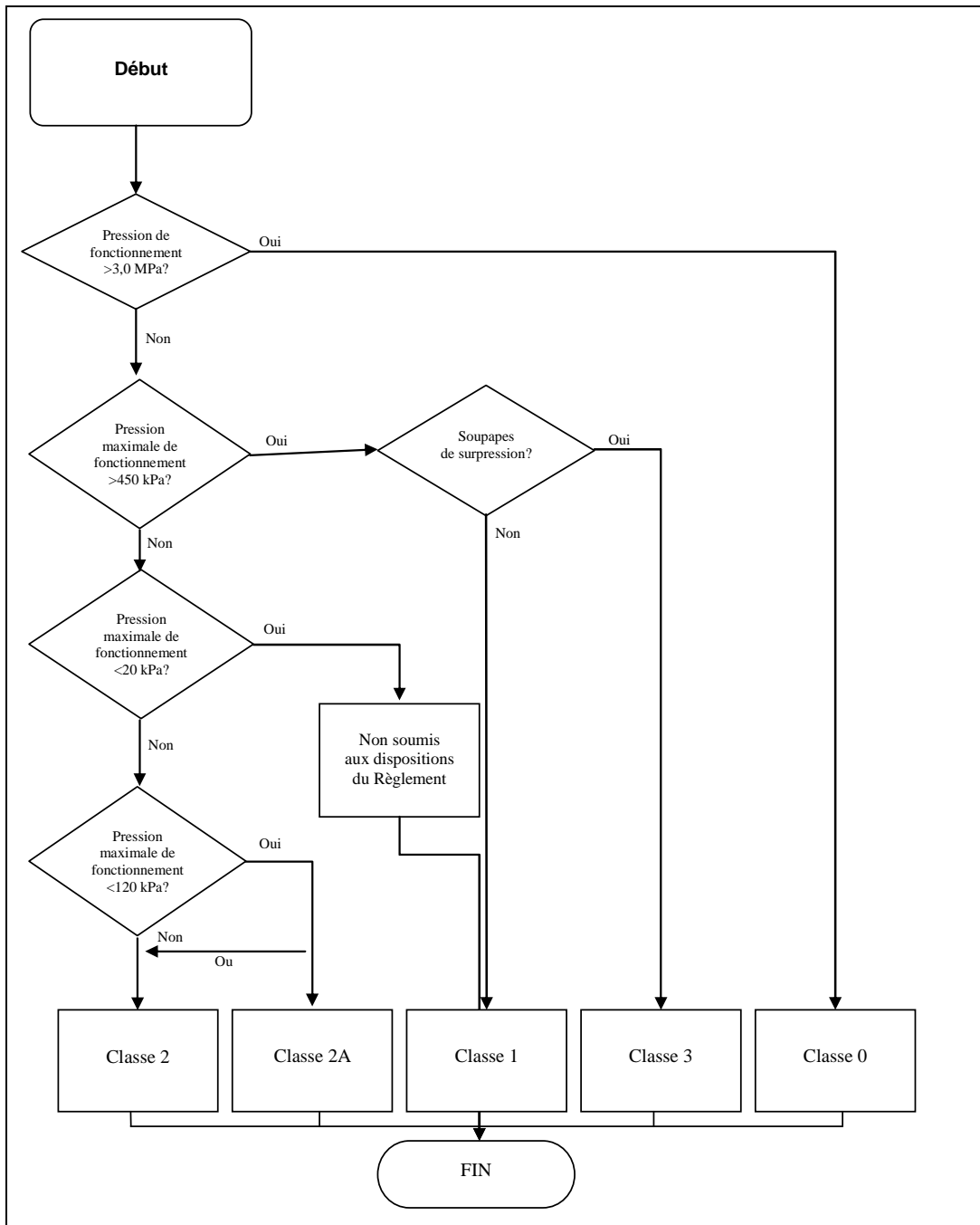
Figure 1 Diagramme de classement des organes en fonction de la pression maximale de fonctionnement et de la fonction
