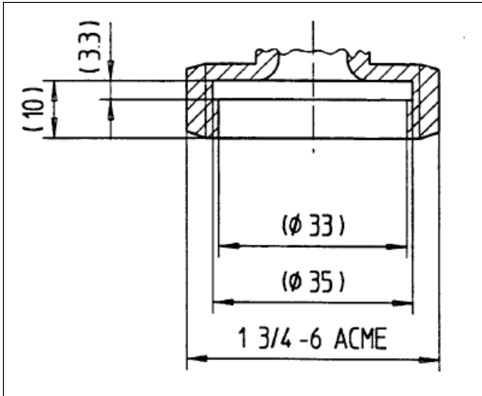
Figure 4 Connecteur de l'embout de remplissage ACME
