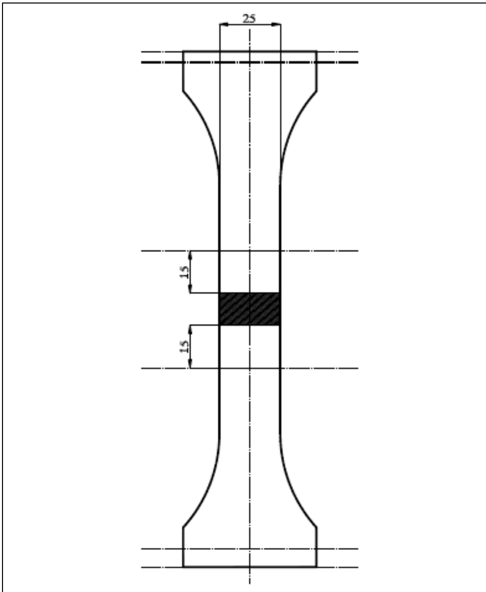
Figure 2 Éprouvette pour l'essai de traction orienté perpendiculairement à la soudure
