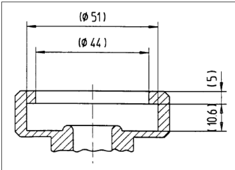
Figure 2 Connecteur de l'embout de remplissage à cuvette
