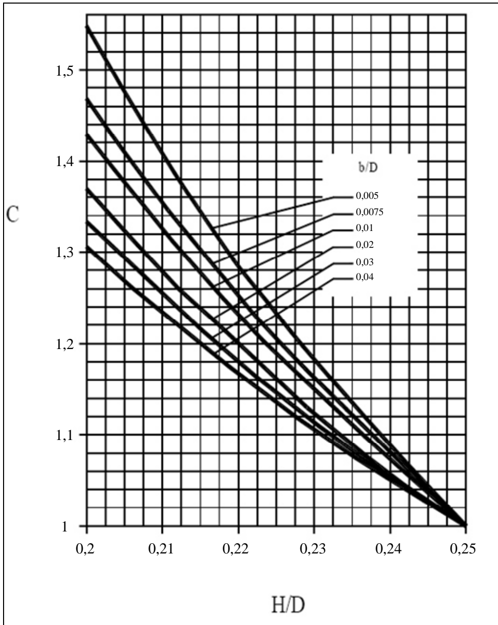
Relation entre le rapport H/D et le coefficient C
