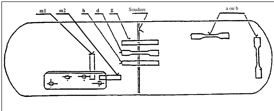
Figure 2a Réservoirs à soudures circulaires uniquement et embase de vanne latérale; emplacement des éprouvettes
