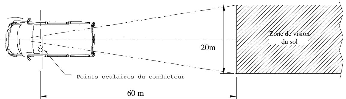
Figure 4 : Champ de vision d'un rétroviseur de la classe I
