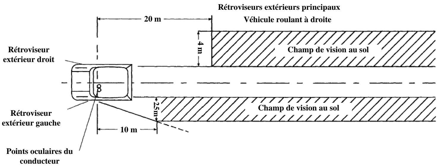
Figure 10: Champ de vision des rétroviseurs de la classe VII.
