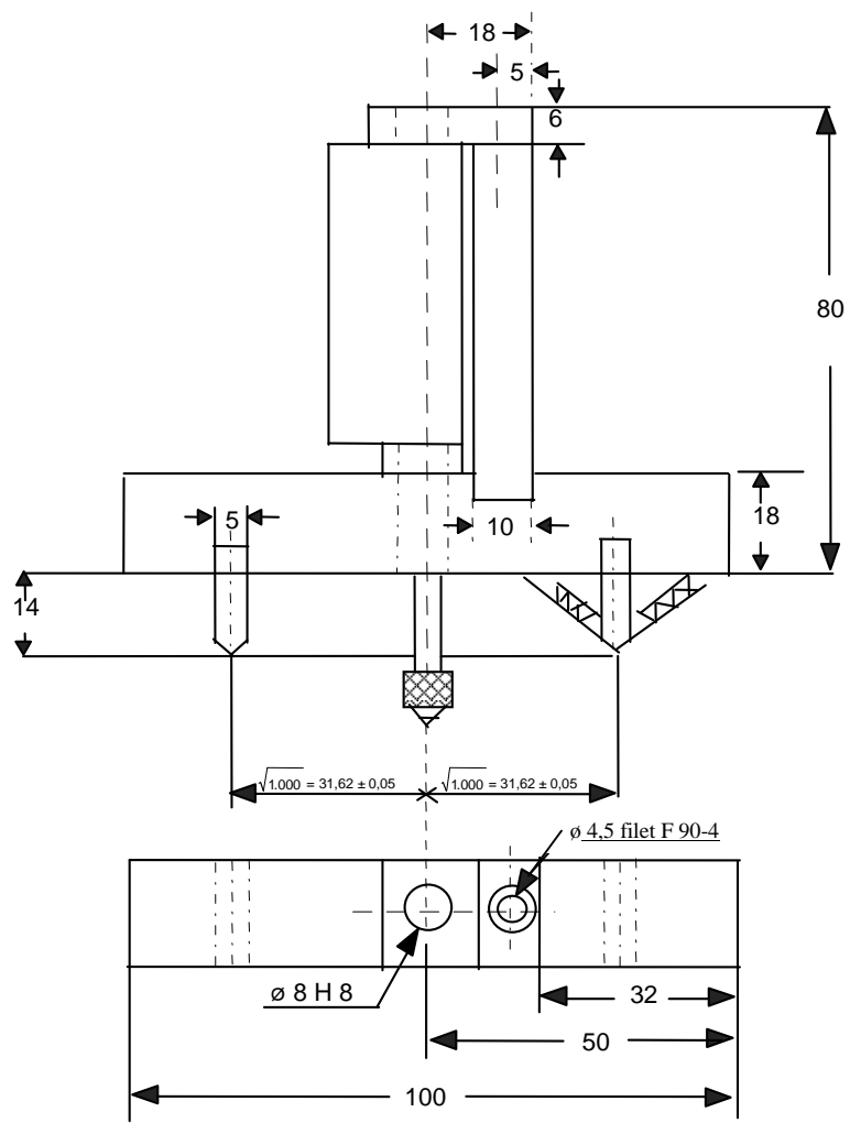
Figure 1: Sphéromètre
