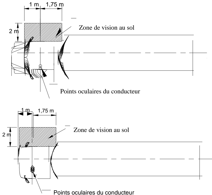
Figures 8a et 8b : Champ de vision d'un rétroviseur «d'accostage» de la classe V
