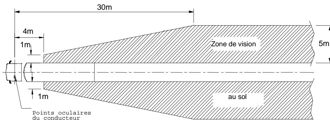
Figure 5 : Champ de vision des rétroviseurs de la classe II
