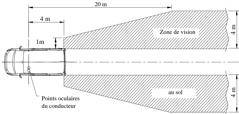
Figure 6 : Champ de vision d'un rétroviseur de la classe III
