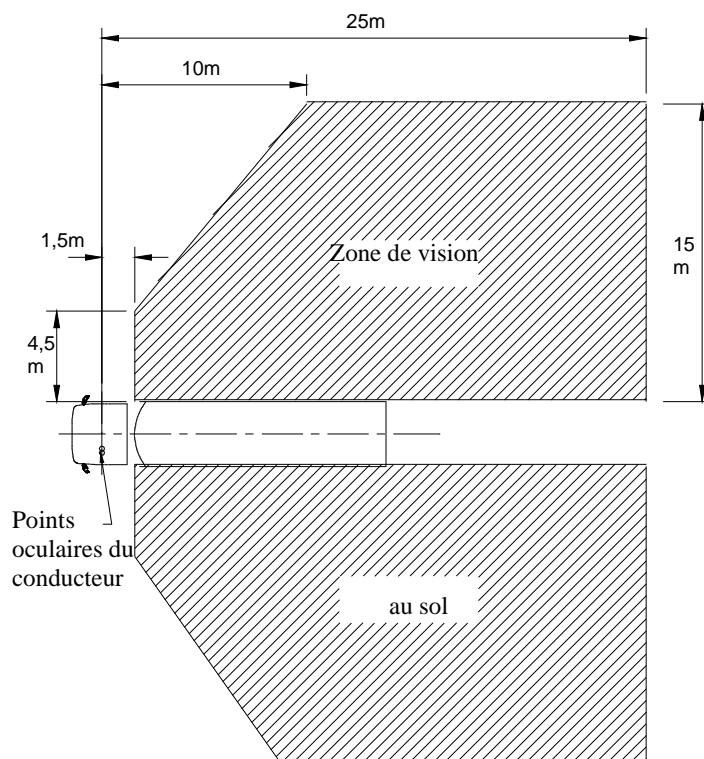
Figure 7 : Champ de vision d'un rétroviseur "grand angle" de la classe IV
