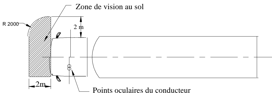
Figure 9: Champ de vision d'un rétroviseur frontal de la classe VI
