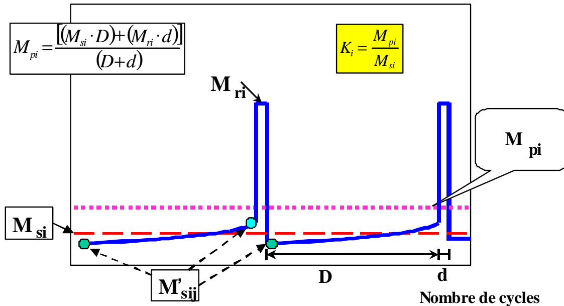
Figure 10/1: Paramètres mesurés lors des essais d'émissions de CO 2 et de consommation de carburant pendant et entre les cycles où se produit une régénération (il s'agit d'un exemple: les émissions pendant la période "D" peuvent en fait augmenter ou diminuer).
