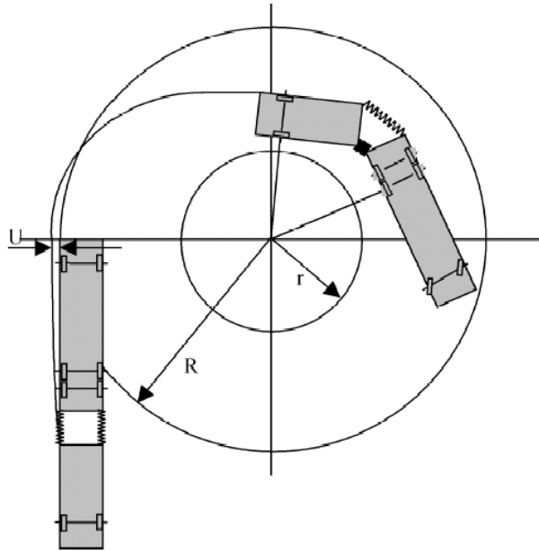
Figure C R = 12,5 \text{ m} r = 5,3 \text{ m} U = 0,6 \text{ m au maximum}
