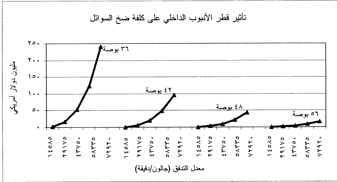
الشكل ١ - أثر قطر أنبوب النقل في كلفة نقل المواد النفطية
