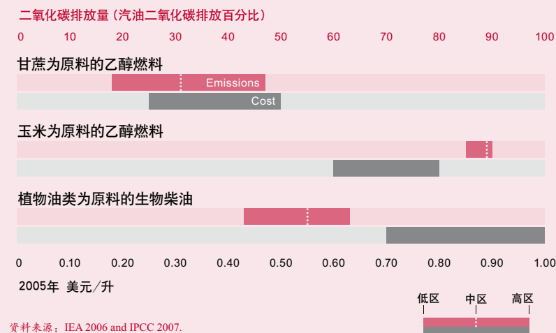
图3.7 生物燃料的成本和减排量各不相同
