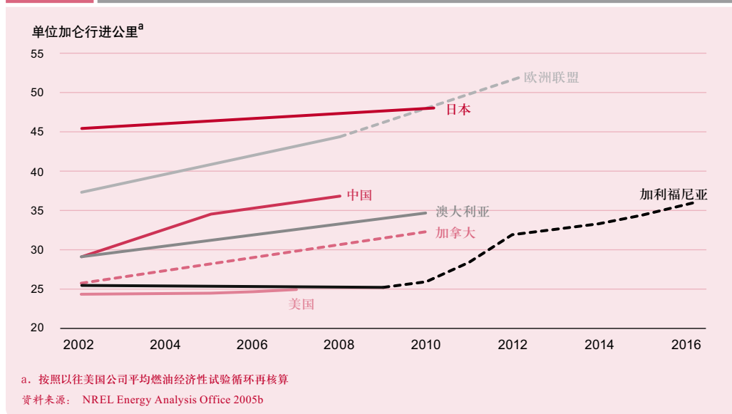
图3.5 富裕国家燃料效率标准各不相同
