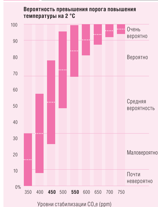
Рисунок 1.9 Риск опасных изменений климата растет по мере увеличения запаса парниковых газов
