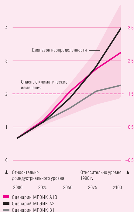
Рисунок 1.2 Глобальный прогноз температуры: три сценария МГЭИК
