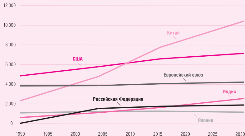
Рисунок 1.15 Выбросы CO 2 , осуществляемые в обычном режиме, имеют тенденцию к росту
