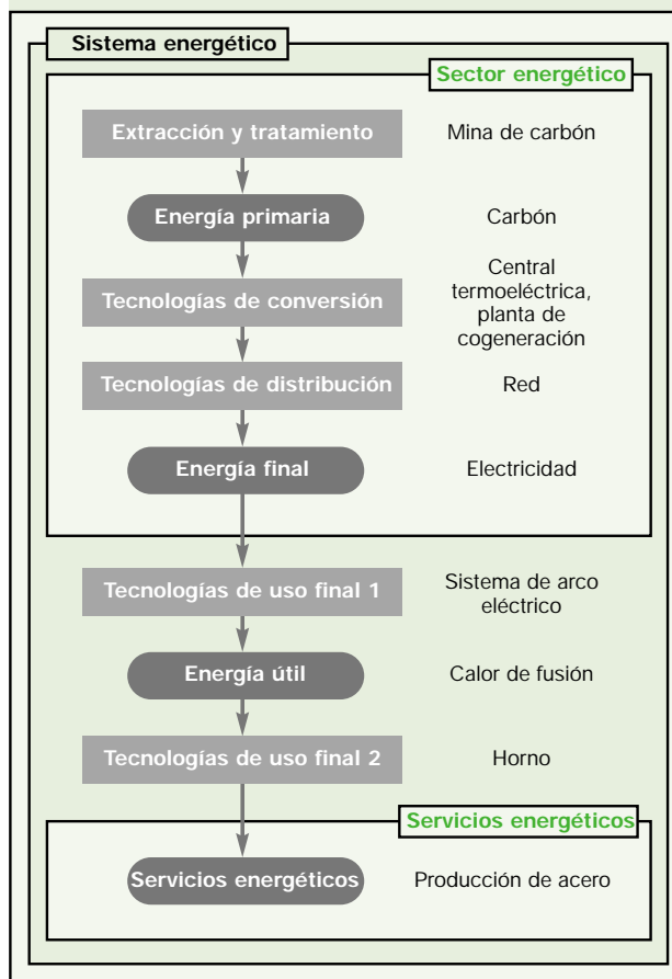
FIGURA 1. UN EJEMPLO DE LA CADENA ENERGÉTICA DESDE LA EXTRACCIÓN A LOS SERVICIOS
