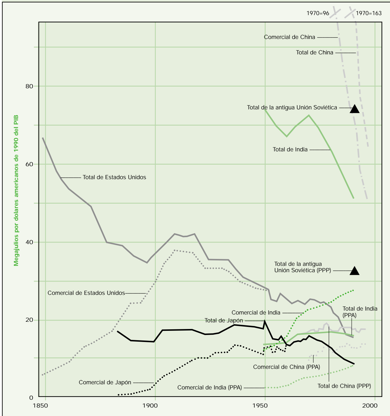
FIGURA 4. TENDENCIAS HISTÓRICAS DE INTENSIDAD ENERGÉTICA PRIMARIA EN LOS DIVERSOS PAÍSES SELECCIONADOS, 1850-2000
