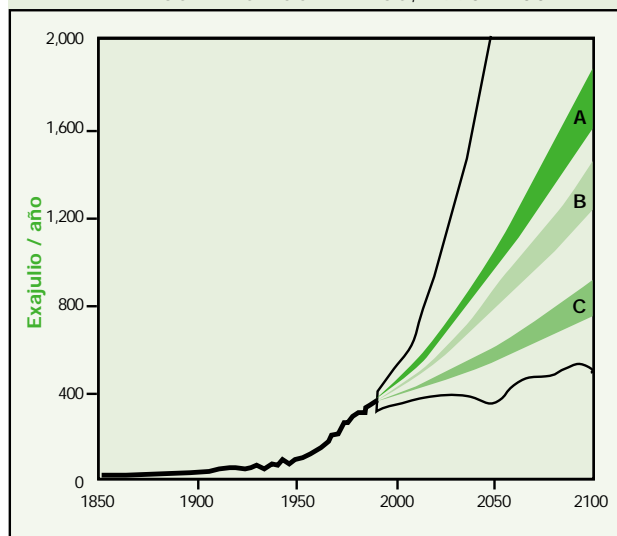
FIGURA 8: REQUISITOS MUNDIALES DE ENERGÍA PRIMARIA COMERCIAL, 1850-1990, Y EN LOS TRES ESCENARIOS, 1990-2100
