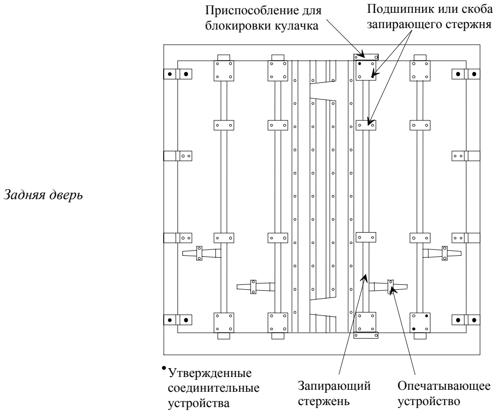
Запорная система двери
