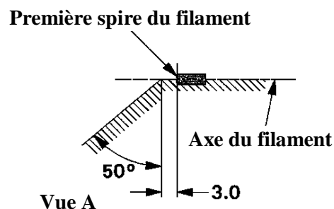
Figure 4. Zone sans partie métallique 6
