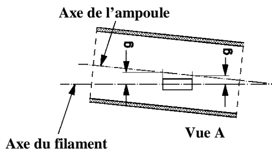
Figure 6. Excentricité de l'ampoule 8
