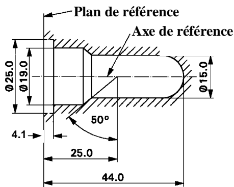
Figure 2. Encombrement maximal 3
