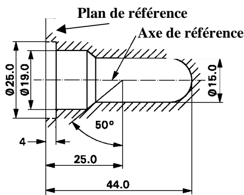
Figure 2. Encombrement maximal 3
