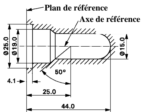
Figure 2. Encombrement maximal³
