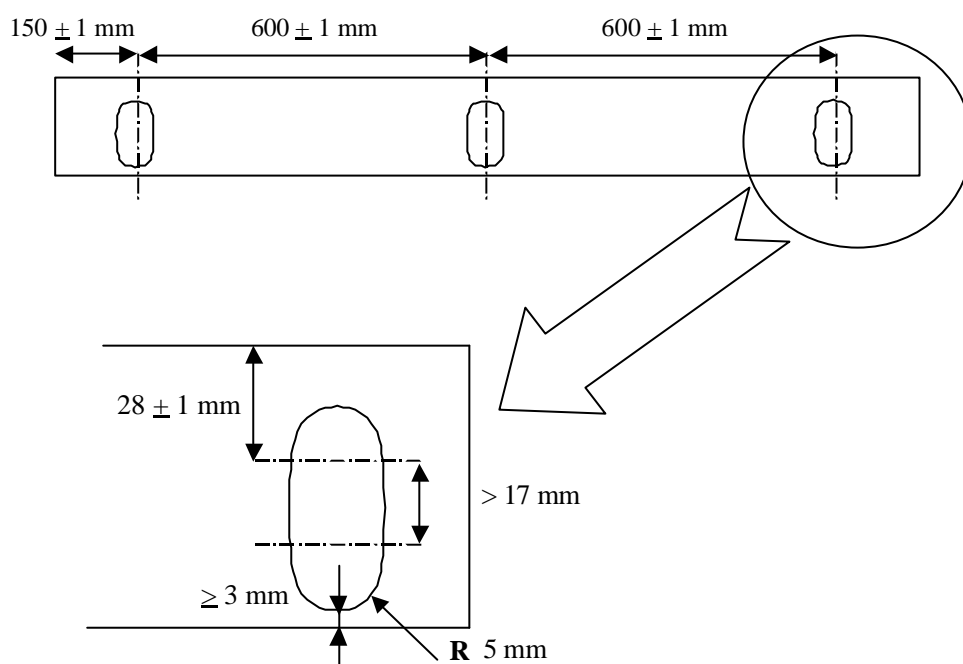
Rebords inférieur et supérieur de la plaque arrière
