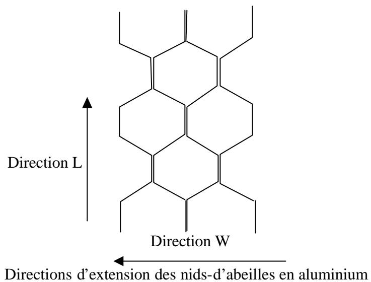
Figure 3. Orientation des nids-d'abeilles en aluminium
