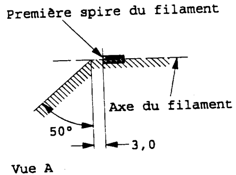
Figure 4 Zone sans partie métallique 8/
