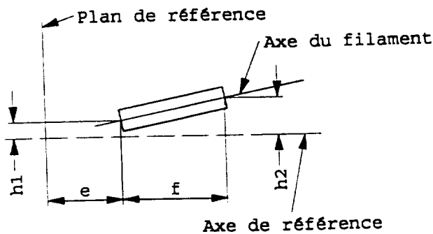
Figure 5 Décalage de l'axe du filament 9/ (lampe à incandescence-étalon seulement)
