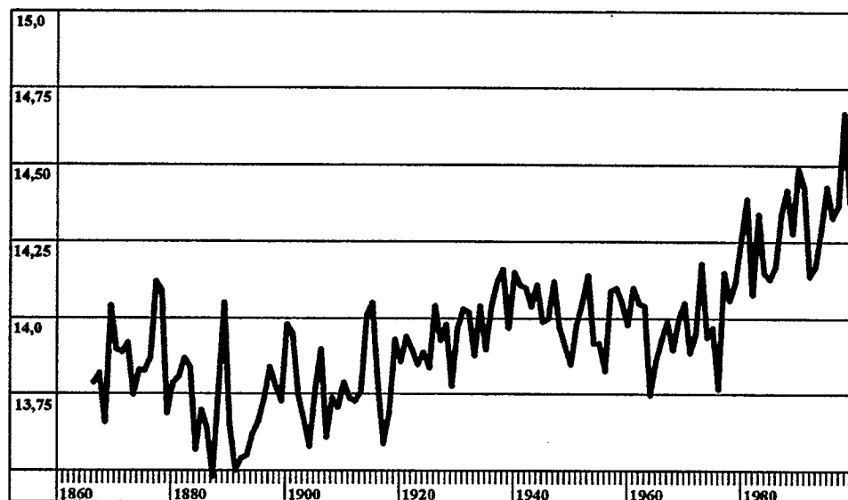
Figure 10 Température moyenne de la surface de la Terre, 1860-1998
