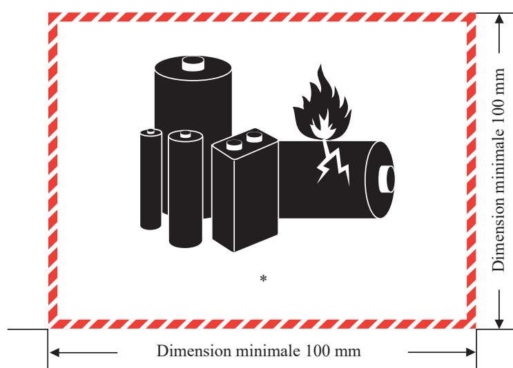
Figure 5.2.1.9.2: Marque pour les batteries
