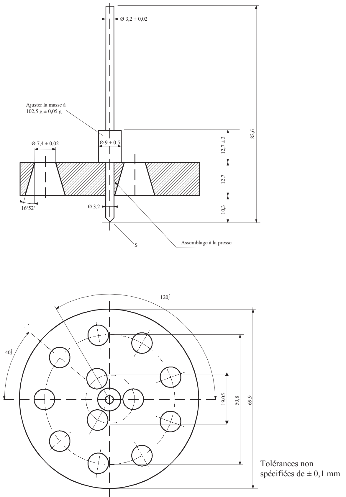
Figure 1 – Pénétromètre
