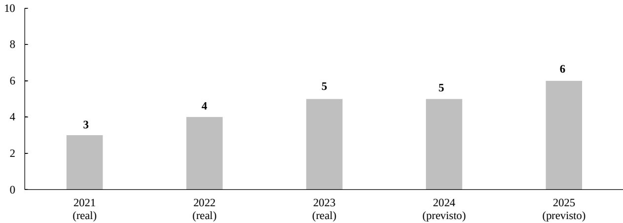
Figura 5.IV Medida de la ejecución: número de satélites lanzados al espacio ultraterrestre a través de la iniciativa Acceso al Espacio para Todos (acumulativo)
