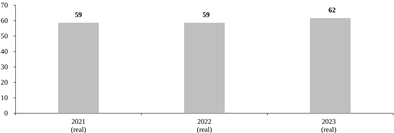
Figura 16.III Medida de la ejecución: número de carreteras designadas autopistas asiáticas en Asia y el Pacífico
