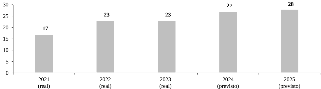
Figura 5.III Medida de la ejecución: número de organismos nacionales de gestión de desastres que pasan a ser usuarios autorizados de la Carta Internacional sobre el Espacio y los Grandes Desastres (acumulativo)
