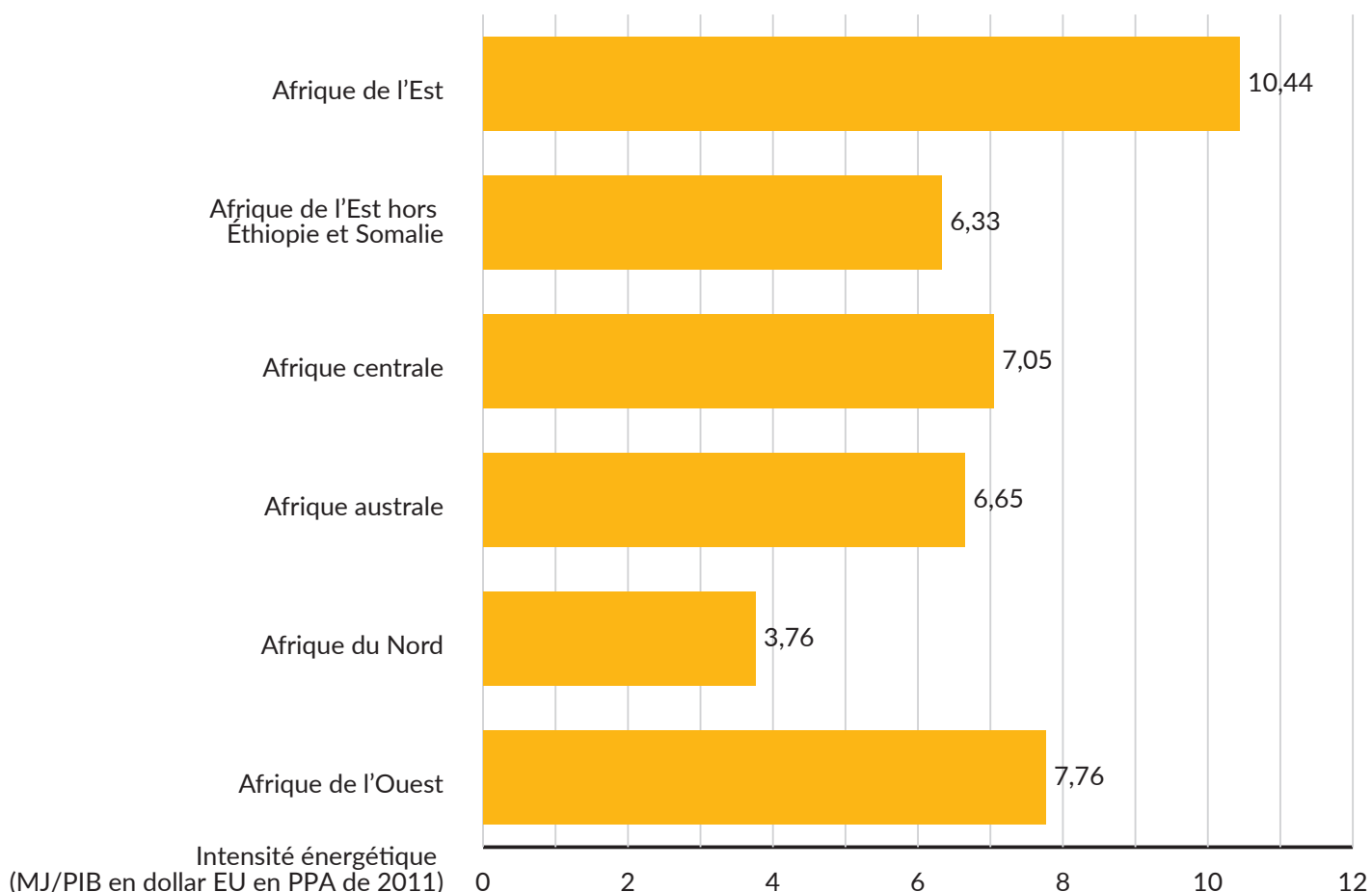
FIGURE 2.7 INTENSITÉ ÉNERGÉTIQUE MOYENNE EN AFRIQUE (MJ/PIB EN DOLLARS EU EN PPA DE 2011) PAR RÉGION, 2015
