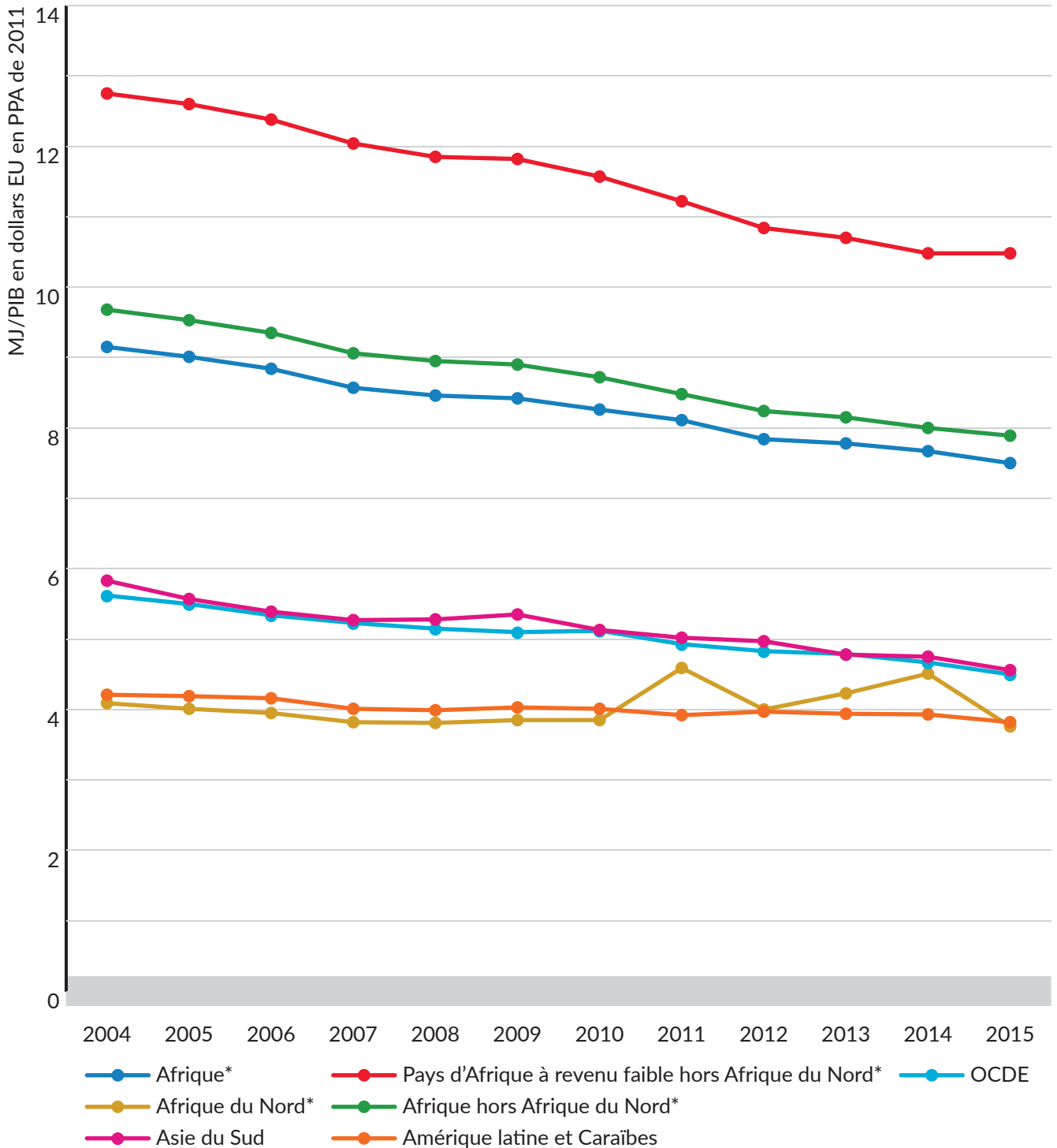
FIGURE 2.6 INTENSITÉ ÉNERGÉTIQUE MESURÉE EN ÉNERGIE PRIMAIRE ET PIB, 2004-2015
