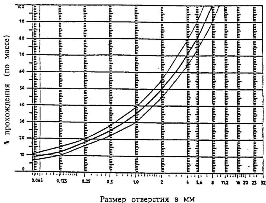
Рис. 2 Гранулометрическая кривая, отражающая состав асфальтобетонной смеси с допусками
