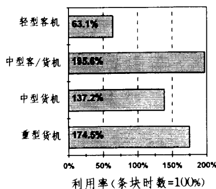
图2. 固定翼飞机利用率(百分比) 1994年6月-9月
