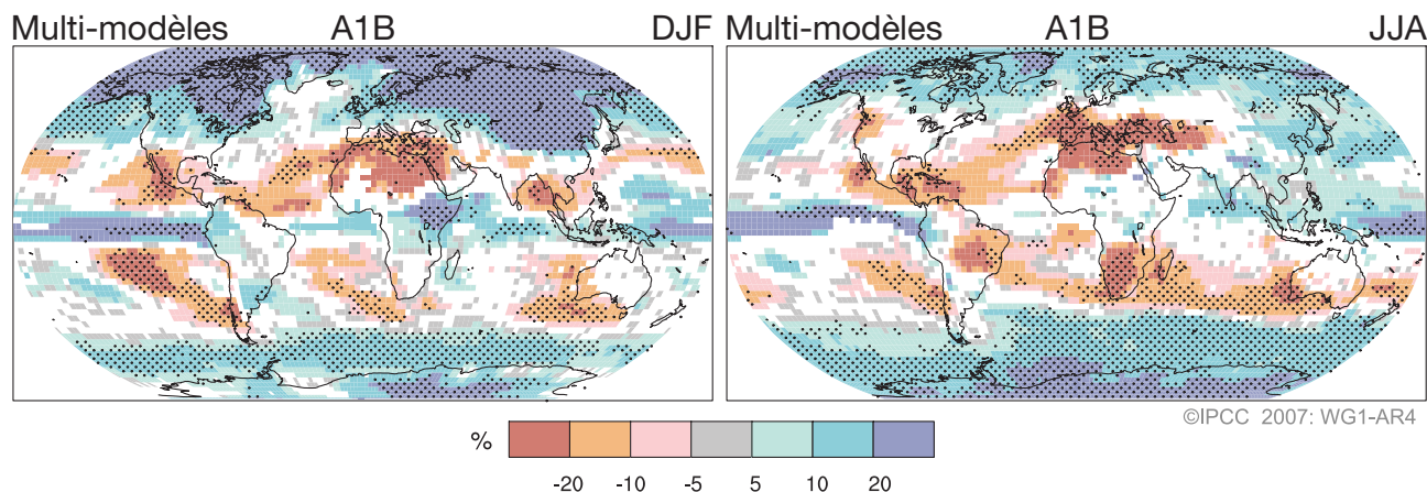
Figure RID.7. Changements relatifs des précipitations (en pourcentages) pour la période 2090-2099 par rapport à 1980-1999. Les valeurs sont issues de moyennes sur de nombreux modèles basés sur le scénario A1B du RSSE pour les mois de décembre à février (à gauche) et de juin à août (à droite). Les aires blanches représentent les zones où moins de 66% des modèles concordent sur le signe du changement, les zones hachurées correspondent aux cas où plus de 90% des modèles concordent sur le signe du changement. {Figure 10.9}
