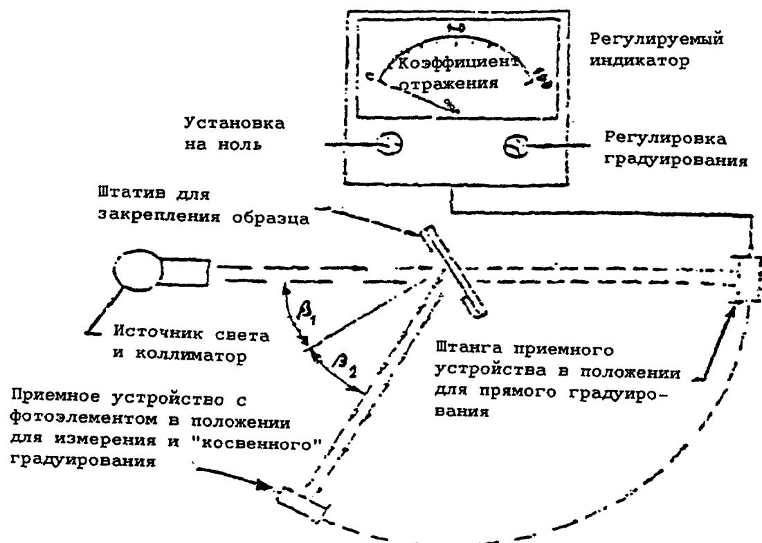
Рис. 1 - Общая схема прибора для измерения отражающей способности двумя методами градуирования
